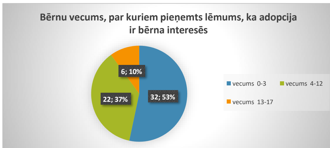
34. diagramma
